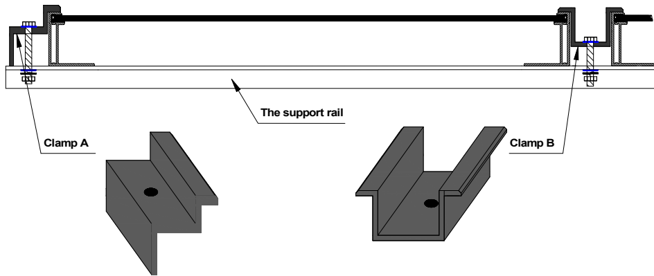
Clamp A: Fasten the Fringe modules
